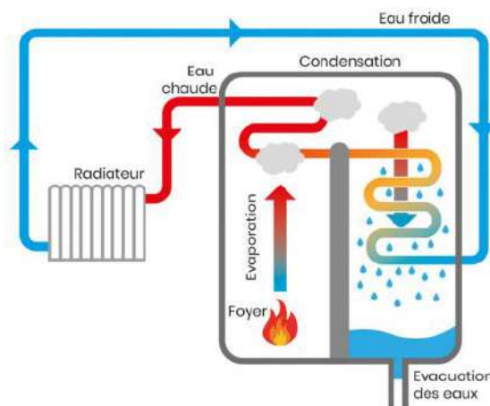
Schéma d'une chaudière à condensation
